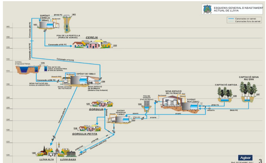
Figura 2 - Esquema vertical de la xarxa actual de Llivia. Font: Agbar
